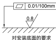
对安装底面的要求
