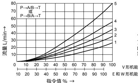
阀的压差为10bar时, 额定流量为25L/min
