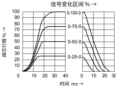
输入信号为阶跃信号时阀的过液性能
