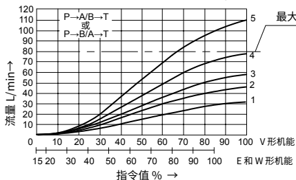
阀的压差为10bar时, 额定流量为32L/min
