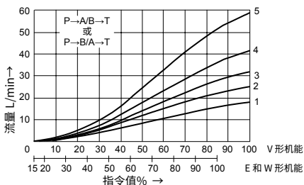
阀的压差为10bar时, 额定流量为16L/min
