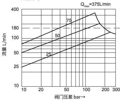
最大容许流量
