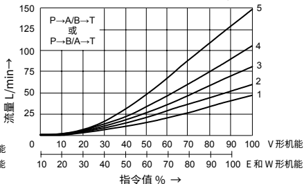
阀的压差为10bar时, 额定流量为50L/min
