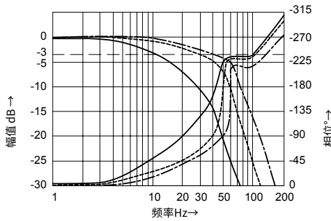
频率响应特性曲线
