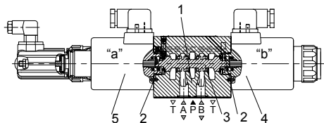
型号 4WRE 10...L2X/...
