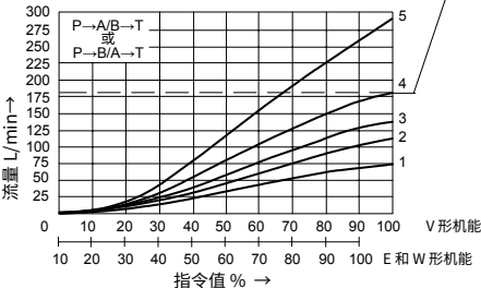
阀的压差为10bar时, 额定流量为75L/min
