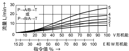
阀的压差为10bar时, 额定流量为8L/min
