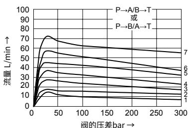
额定流量为 60 L/min 的功率极限
